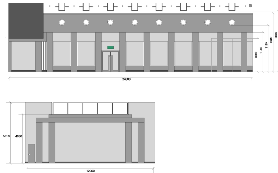
側面図
